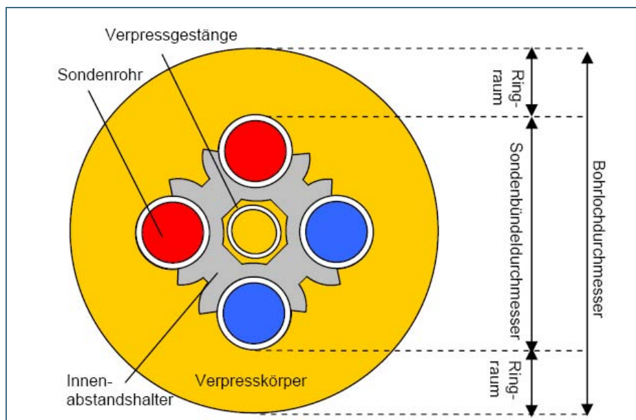
Abb. 2: Systemschnitt Erdwärmesonde: Bohrdurchmesser in Abhängigkeit vom Ringraum und Sondenbündel (LfU, Berger)
